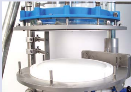
Filter plate with lowering device for easy filter change Filterplatte mit Absenkvorrichtung für einfachen Filterwechsel
