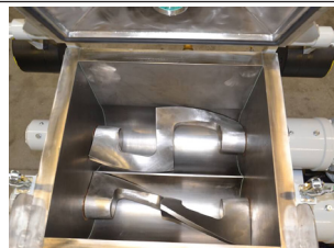
Z-BLANDARE/KNÅDARE
