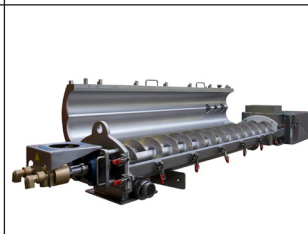
VÄRME-/KYLSCRUVAR
