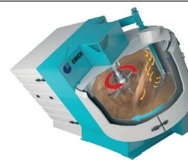
BLANDNING/GRANULERING
